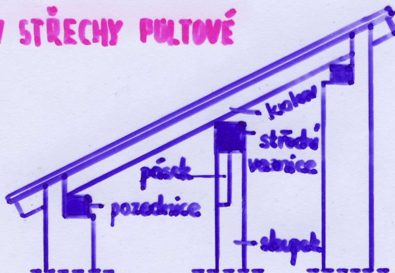
SVISLÝ ŘEZ
