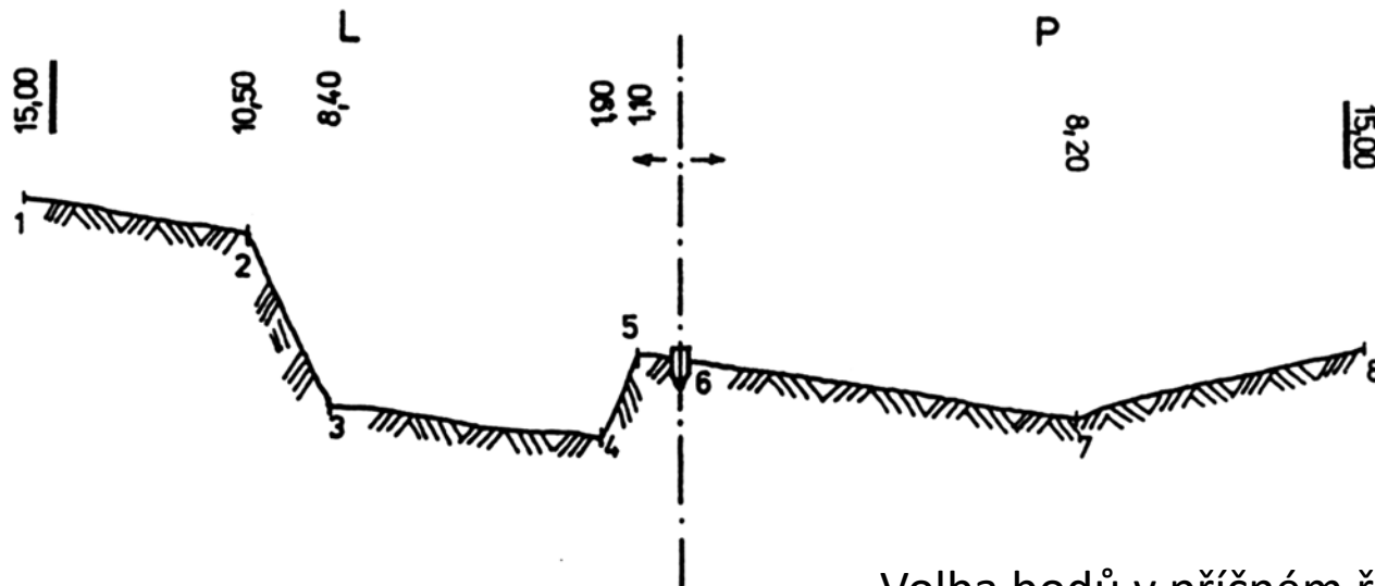
Volba bodů v příčném řezu
